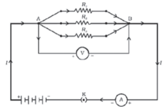
चित्र 11.7 अवरोधहरूको समानान्तर जडान
